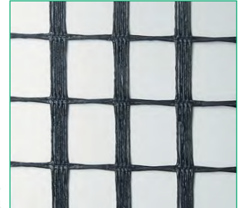
Fig. 3 Knitted/woven geogrid
